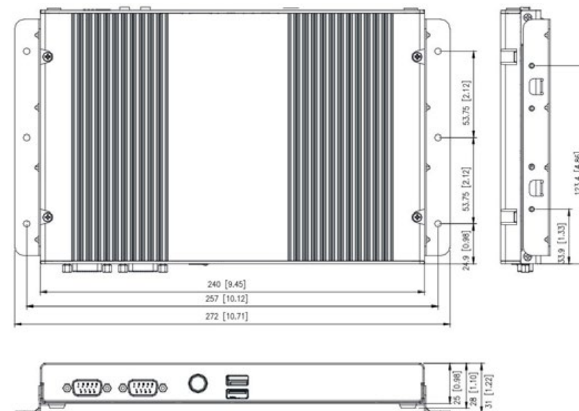
Dimensiones en mm y [pulgadas]
