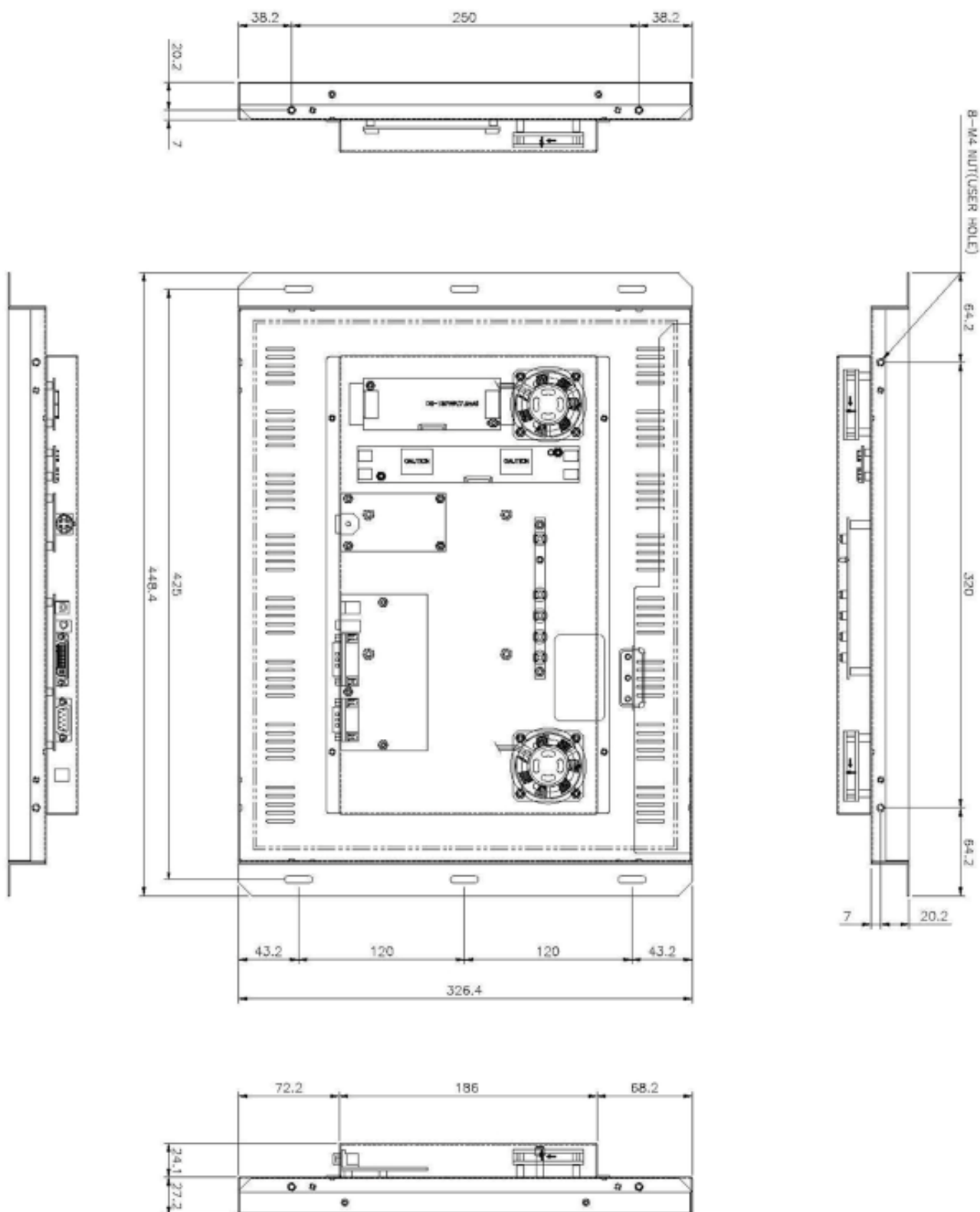
Dimensiones del monitor SV-LM190K HB en mm
